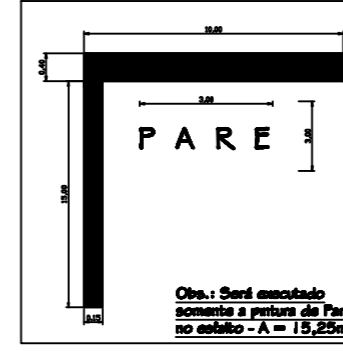
● DETALHE DA SINALIZAÇÃO DE PARE (45 X)
